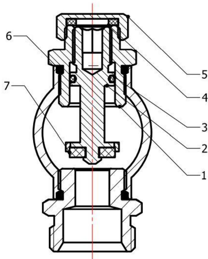
Рис. 1. Устройство подающей гребенки без ротаметров
