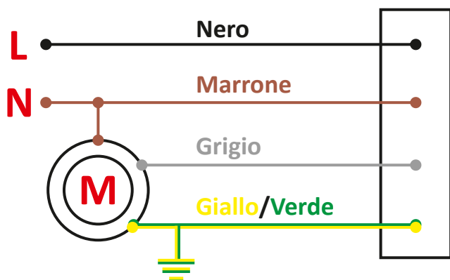
Collegamento senza spina
