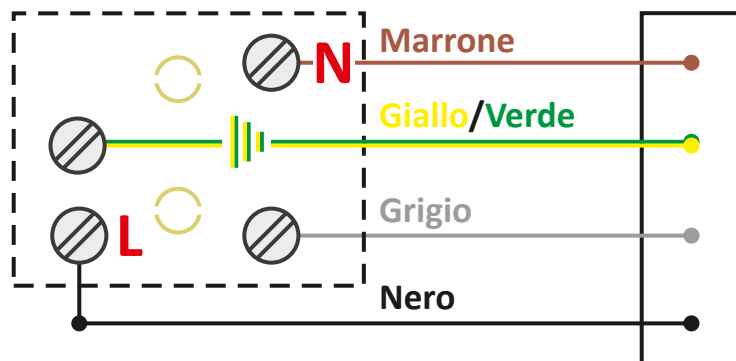
Collegamento con spina intermedia Schuko
