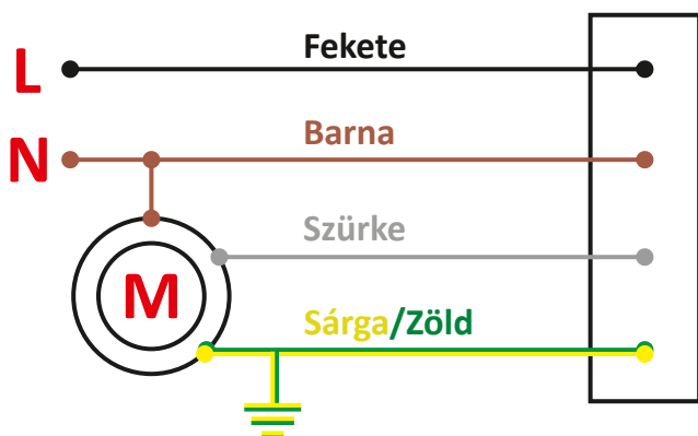
Csatlakozó nélküli csatlakozás
