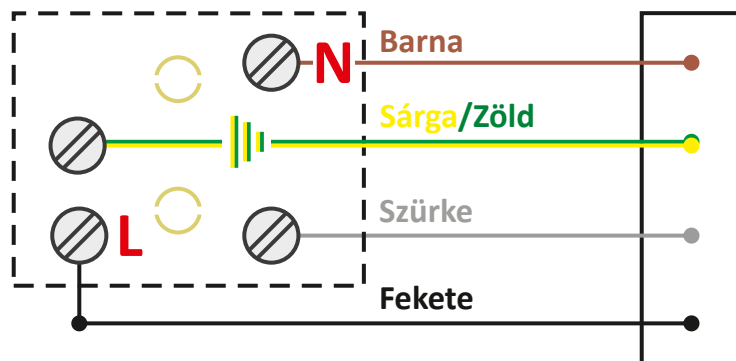
Csatlakozás Schuko köztes csatlakozóval
