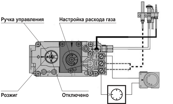
Рисунок 11 Схема подключения комнатного термостата
