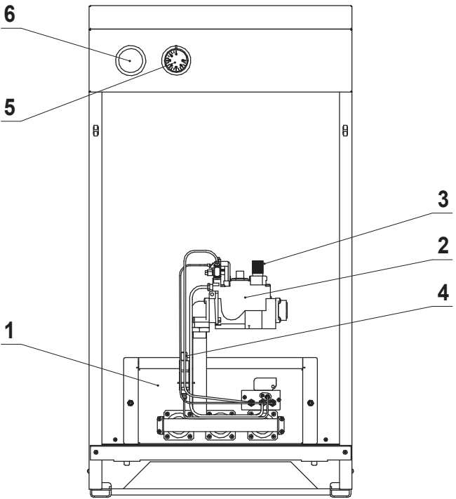
Рисунок 2 Конструкция котла с газовым блоком SIT 820 mV 1) газогорелочное устройство ГГУ; 2) газовый блок; 3) ручка управления газовым блоком; 4) кнопка пьезорозжига; 5) ручка терморегулятора; 6) термометр; 7) дымосборник; 8) датчик тяги; 9) теплообменник с топкой; 10) горелка; 11) теплоизоляция; 12) гильза; 13) турбулизатор; 14) датчик перегрева теплоносителя.
