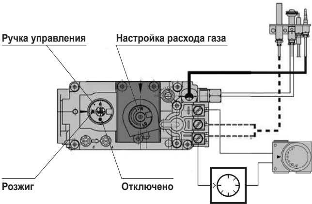
Рисунок 11 Схема подключения комнатного термостата
