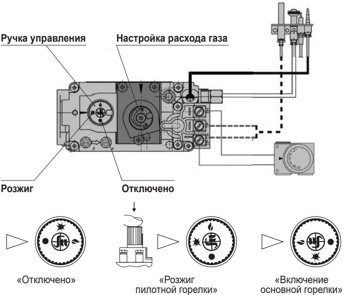
Рисунок 10 Элементы управления и регулировки на газовом блоке
