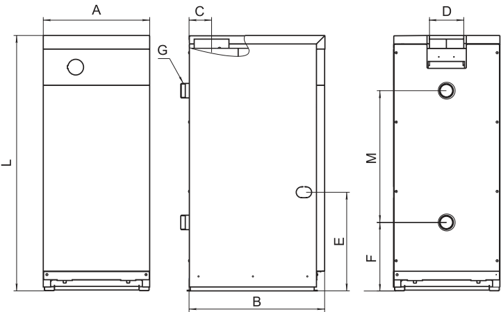
Рисунок 1 Общий вид, габаритные и присоединительные размеры котлов
