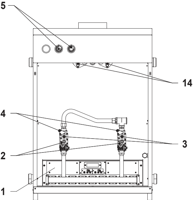
Рисунок 3 Особенности котла TORINO-100 с двумя газовыми блоками 820 NOVA mV
