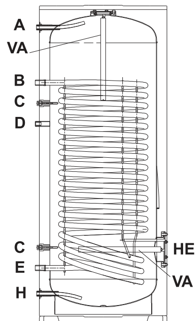
ECOUNIT 100/150/200/300 L-1C
