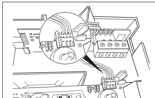
Sl. 4.1 Prikllop vodila na priključno sponko v grelniku
