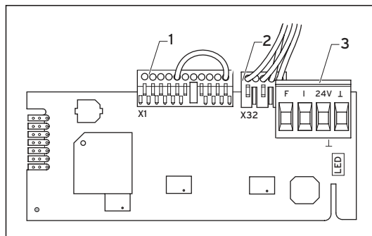
Sl. 3.4 Priključci kod zadane vrijednosti temperature polaznog voda (s utikačem X1)
