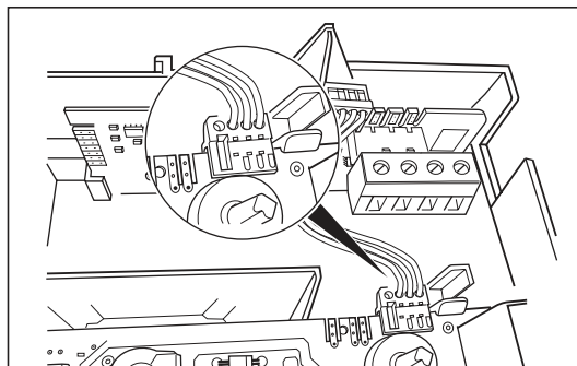
Рис. 4.1 Підключення дроту шини до з'єднувальної клемки опалювального приладу
