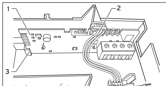
Sl. 4.2 Vgradnja ploščice tiskanege vezja vmesnika 0-10 V
