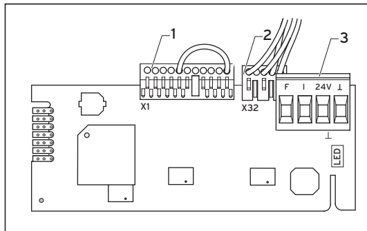
Şekil. 3.4 Kablo bağlantıları (soketli X1)
