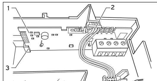
Sl. 4.2 Ugradnja elektroničke ploče sučelja 0-10 V
