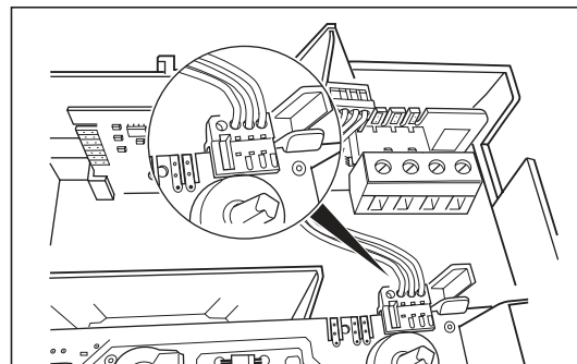
Sl. 4.1 Spajanje sabirničkog voda na priključnu stezaljku u uređaju za grijanje
