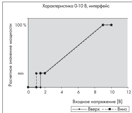
Рис. 3.1 Характеристика интерфейса O-10 B с расчетным значением мощности
