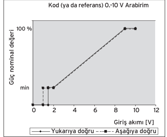
Şekil. 3.1 Güç - giriş akımı 0-10 V karakteristik eğrisi
