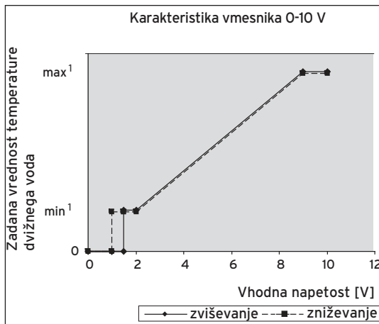
Sl. 3.2 Karakteristika vmesnika 0-10 V z zadano vrednostjo temperature dviznega voda
