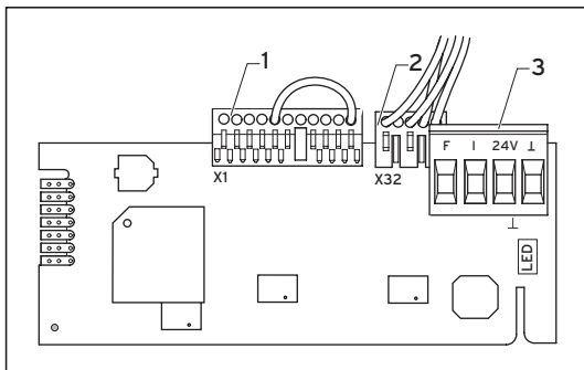
Obr. 3.4 Prípojky pri požadovanej hodnote prírodnej teploty (so zástrčkou X1)
