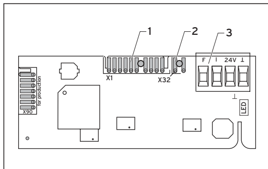
Sl. 3.3 Priključci kod zadane vrijednosti snage (bez utikača X1)
