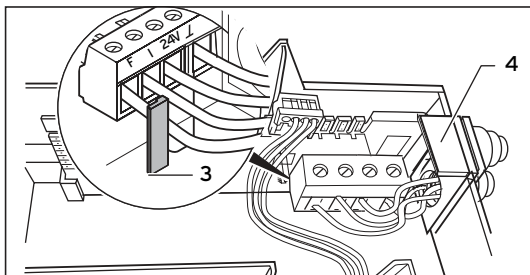
Şekil. 4.3 Kablo tutucu
