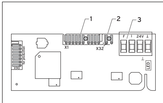
Sl. 3.3 Priključki pri zadani vrednosti moči (brez vtiča X1)
