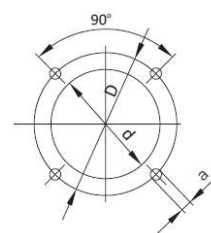
Размеры фланца
