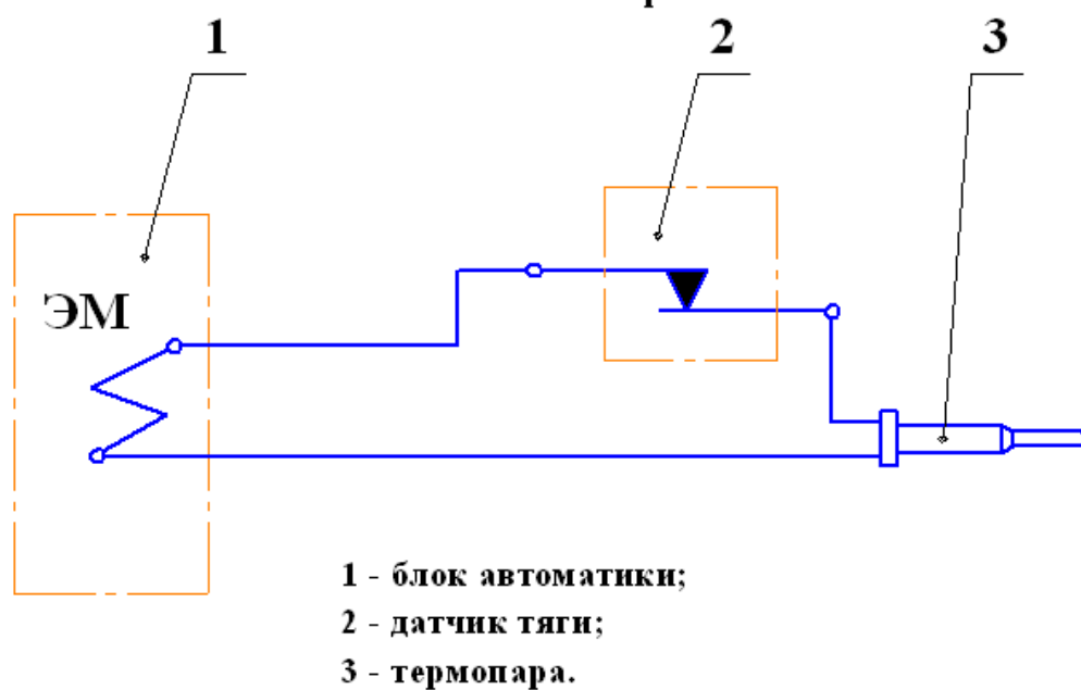
Рис.3 Схема электрическая.
