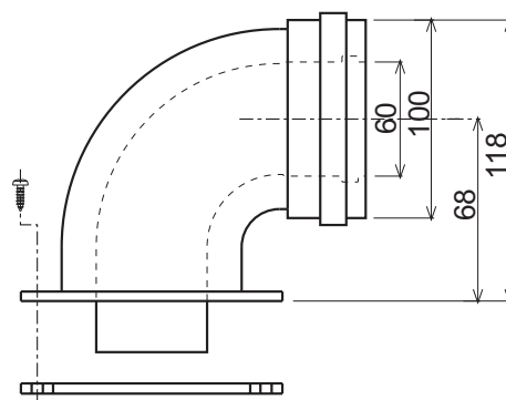
рис. 13 - Элементы для коаксиальных воздухопроводов
