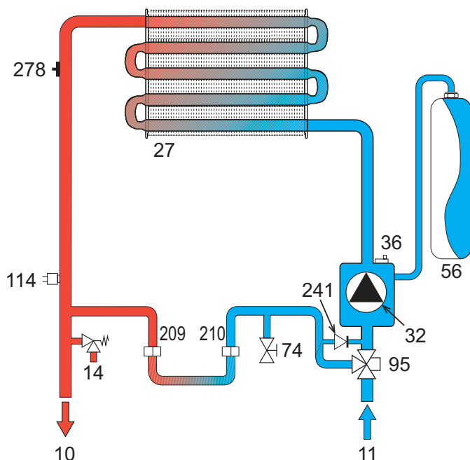
рис. 29- Контур отопления
