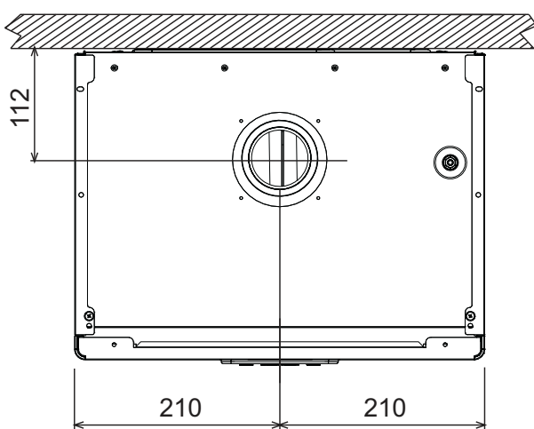
рис. 60- Вид сверху
