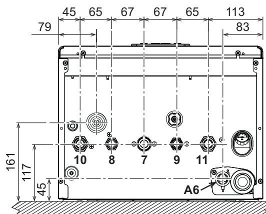
рис. 61- Вид снизу
