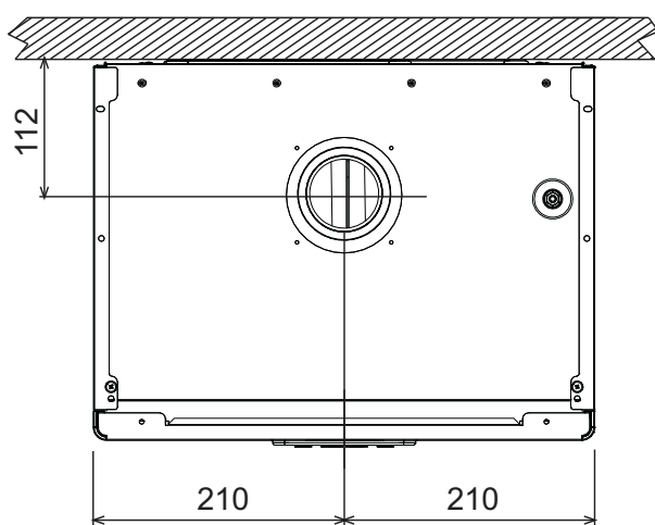
рис. 60- Вид сверху
