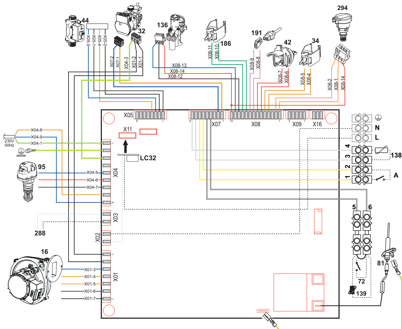
рис. 67- Электрическая схема
