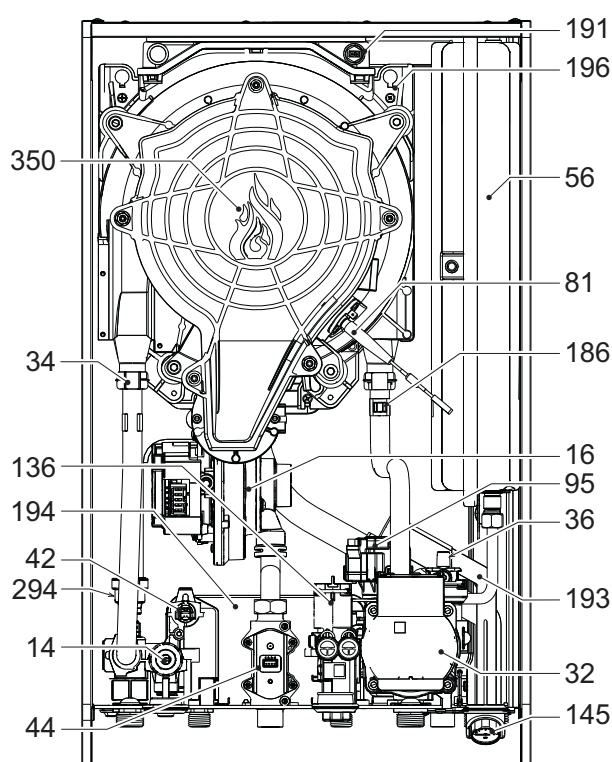
рис. 62- Общий вид
