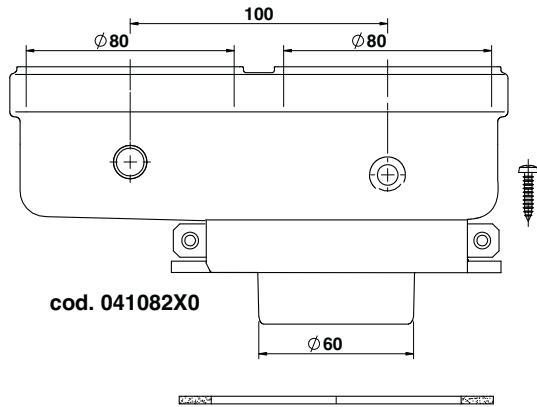
рис. 33- Исходная принадлежность для отдельных труб
