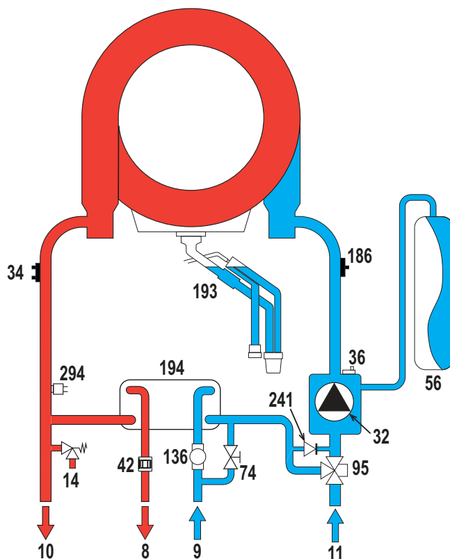
рис. 63- Гидравлический контур
