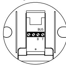
Klemmenstrook Bus van de Eenheid Klemmenstrook van de afstandbediening
