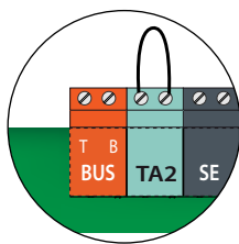
Bornier Bus de la Chaudière
