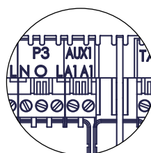
Morsettiera dell'interfaccia di sistema
