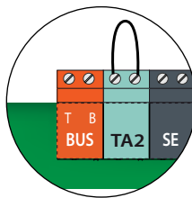
Terminal BUS de la caldera
