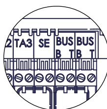
Klemmenstrook Bus van de Eenheid
