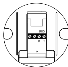
Контактная колодка дистанционного управления блока
