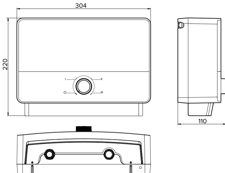
AURES M 10.5 - AURES M 12
