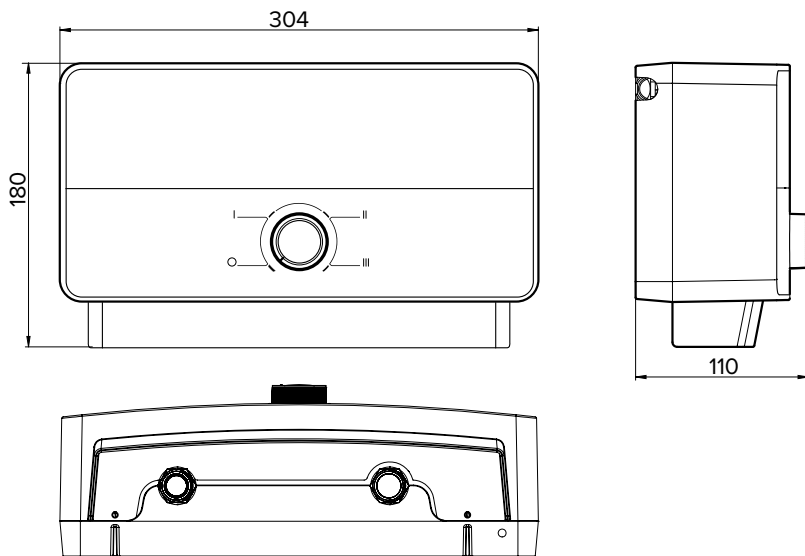
AURES M 6 - AURES M 7.7 - AURES M 8
