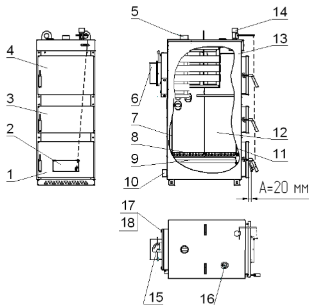
Рис.2 Котлы KC-T...-20-20p; KC-T...-30-30p; KC-T...-40-40p
