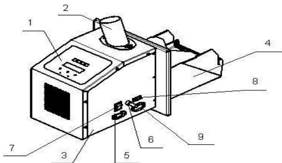
Рис. 31 Пеллетная горелка
