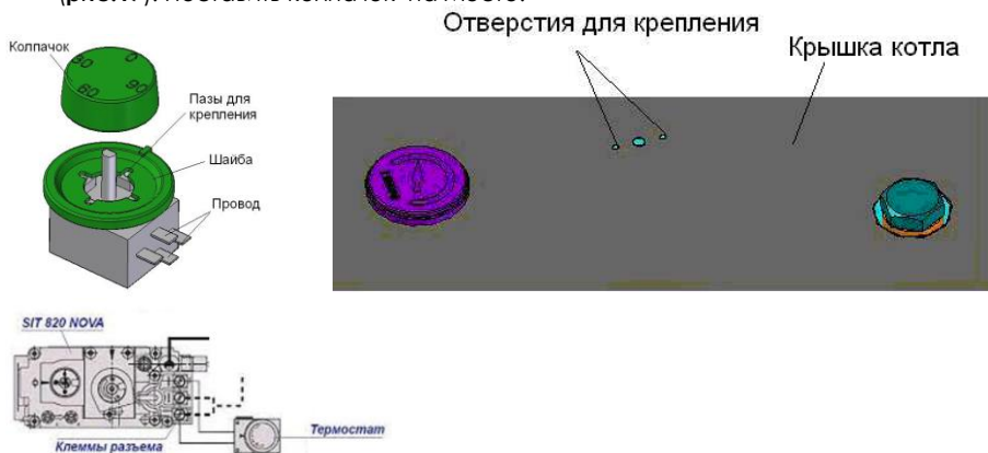
Рис.18 Установка и соединение термостата капиллярного.
