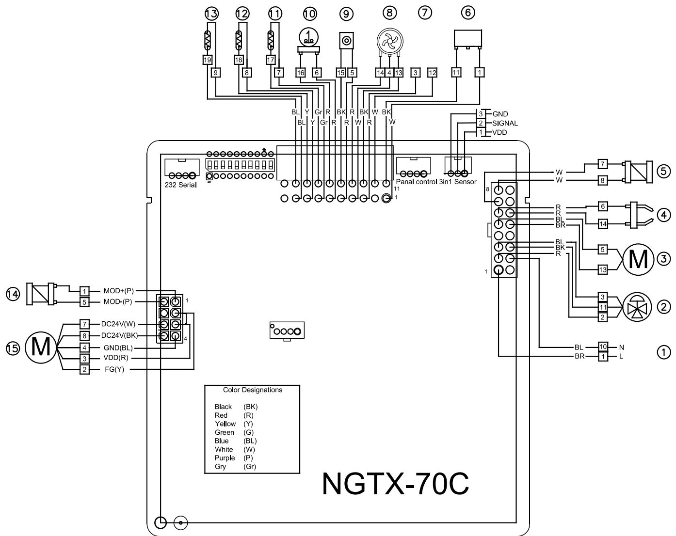
Рисунок 14. Схема электрическая.
