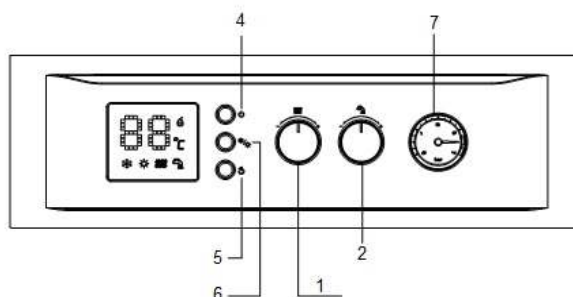
Котлы C32F-C40F
