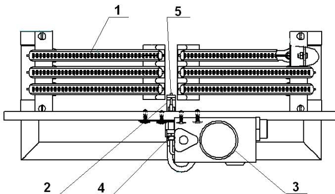
рис.2 Горелка УГ-...
