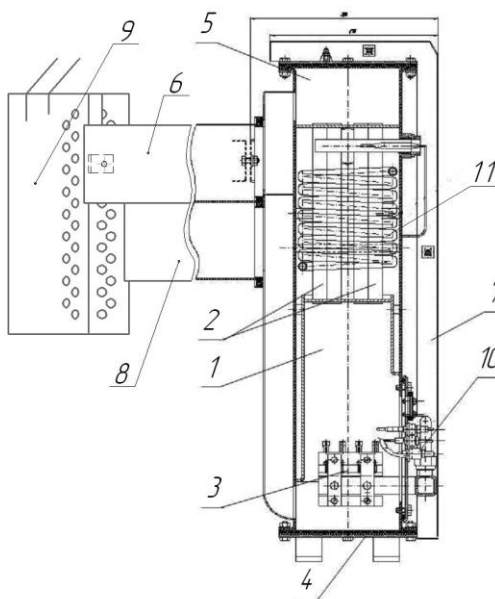
Рис. 1 – Котёл отопительный газовый КС-Г/ГВ ...- П
