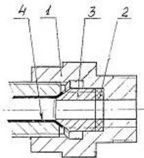
Рис. 4 – Переходной штуцер.
