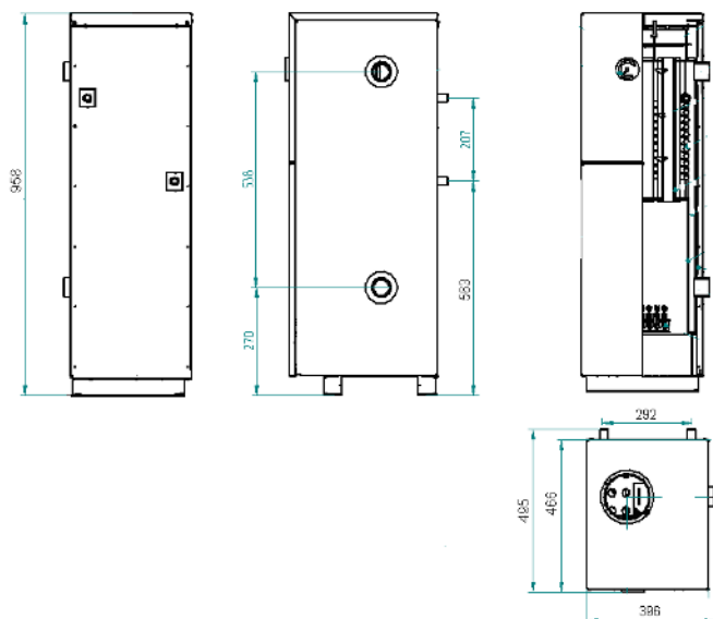
рис. 3 Аппараты АОГВ/АОГБК -17,4-1; АОГВ/АОГБК -17,4Т-1. Остальное см рис. 1
