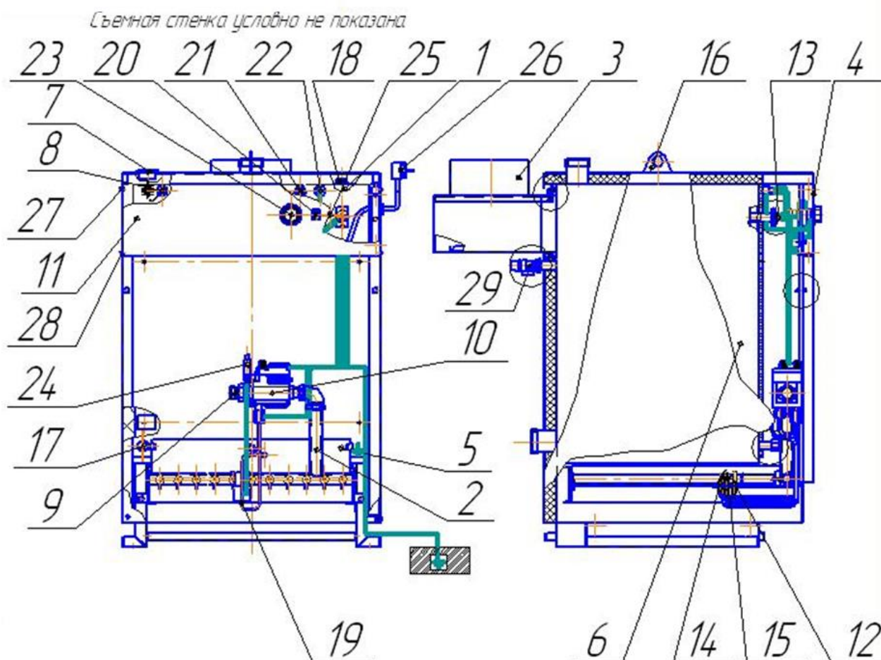
Рис.2 Конструкция котла
