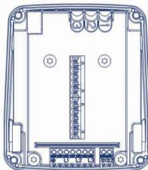
Abbildung 5: Elektronik ohne Kippschalter.
