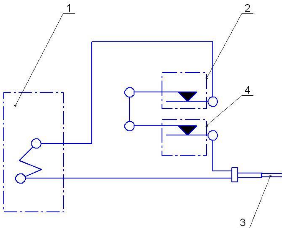
Рис.3 Схема электрическая.
