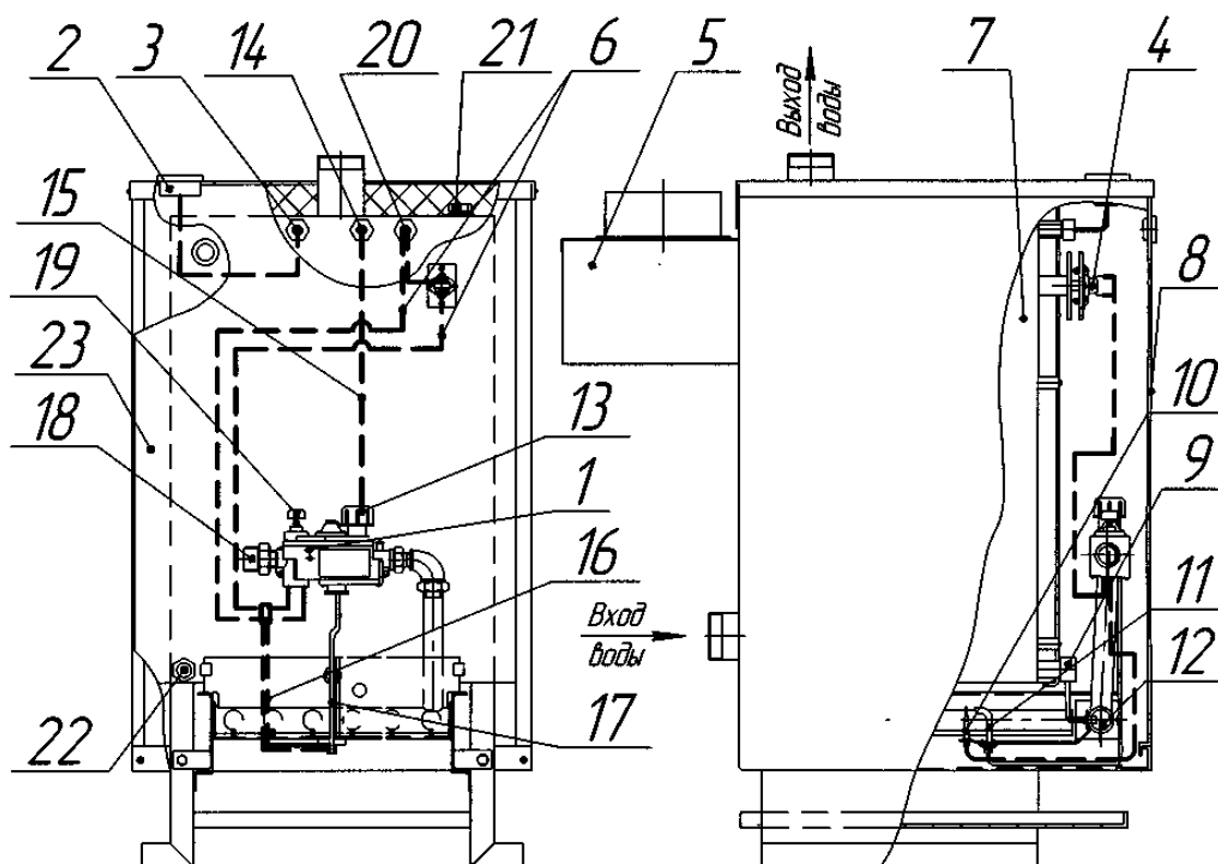
Рис. 2. Конструкция котла.
