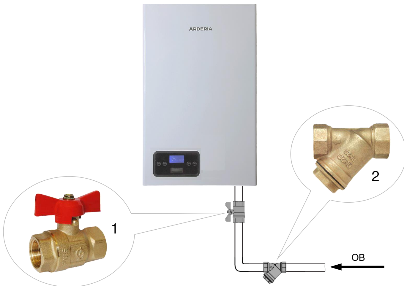
Рис. 18 Монтаж труб системы отопления 1. запорный кран; 2. косой фильтр «грязевик»
