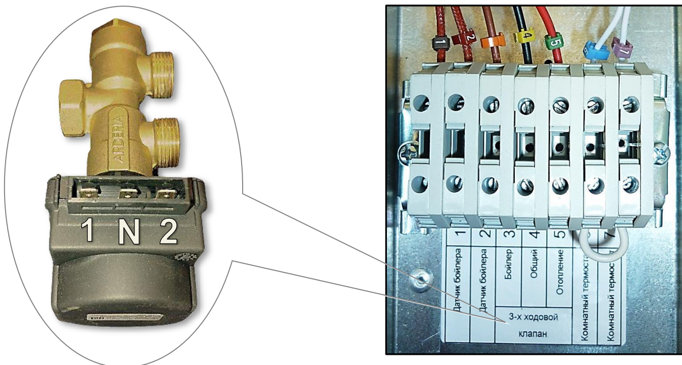
Рис.22 Подключение трехходового клапана «ARDERIA» к клеммной колодке.
