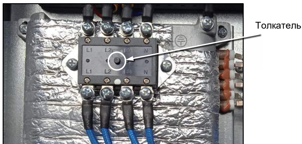
Рис. 8 Силовой биметаллический термостат (датчик перегрева)
