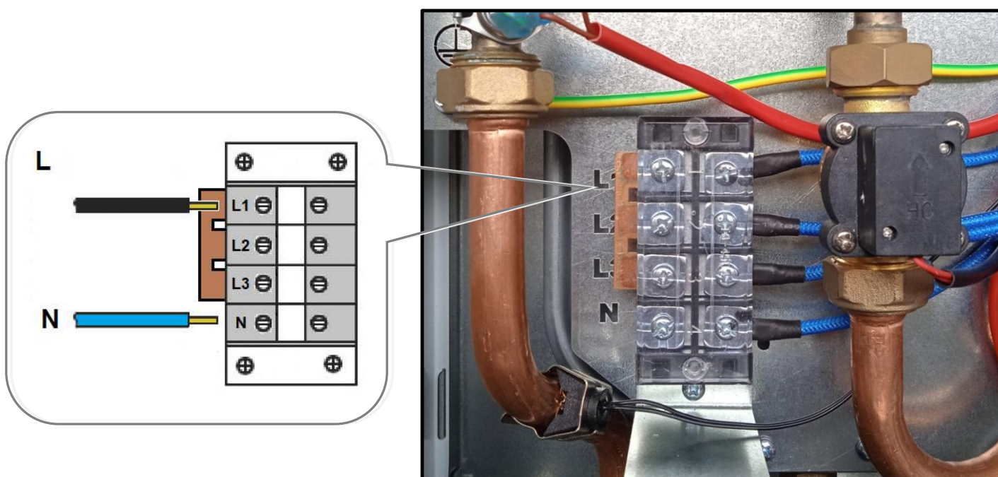
Рис. 15 Однофазное подключение
