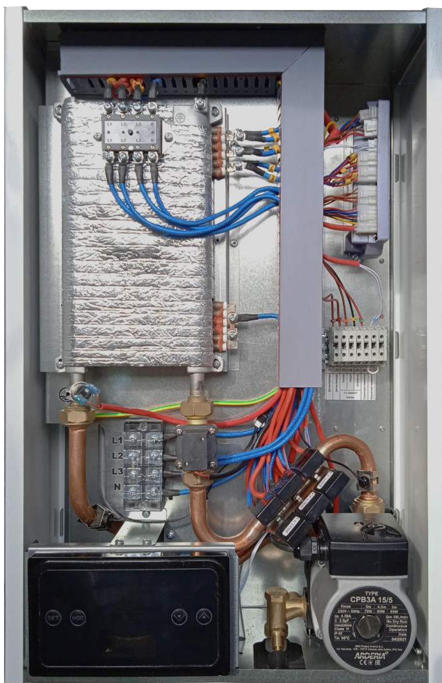
Рис. 1 Общий вид
