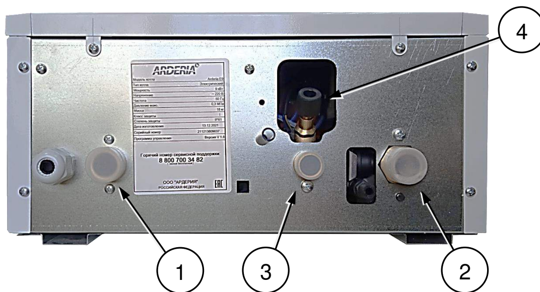
Рис. 17 Патрубки присоединения электрокотла к трубам 1. выход ОВ из электрокотла «подача»; 2. вход ОВ в электрокотёл «обратка»; 3. вход ХВС в электрокотёл; 4. кран подпитки
