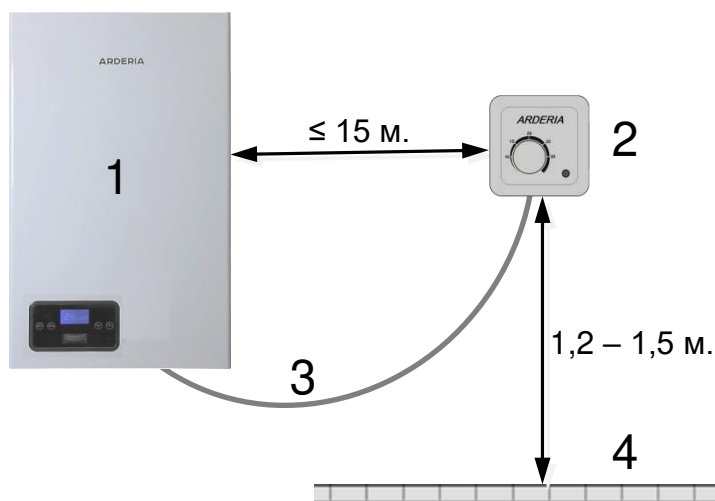
Рис. 20 Место установки комнатного термостата
