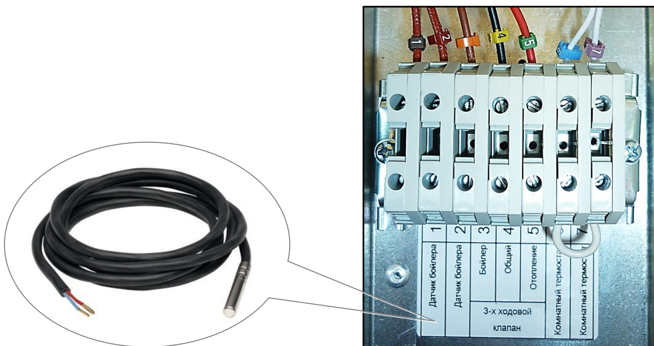
Рис.23 Подключение датчика температуры бойлера трехходового клапана «ARDERIA» к клеммной колодке.
