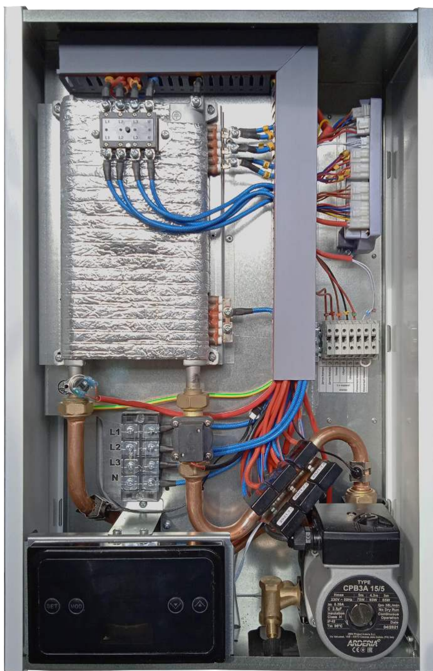
Рис. 1 Общий вид
