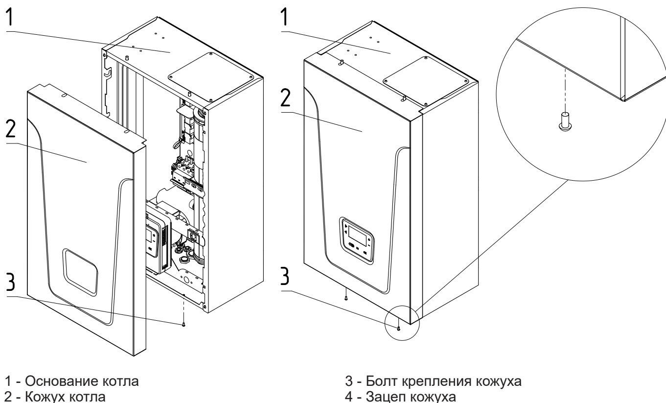
Рис.7 Снятие кожуха
