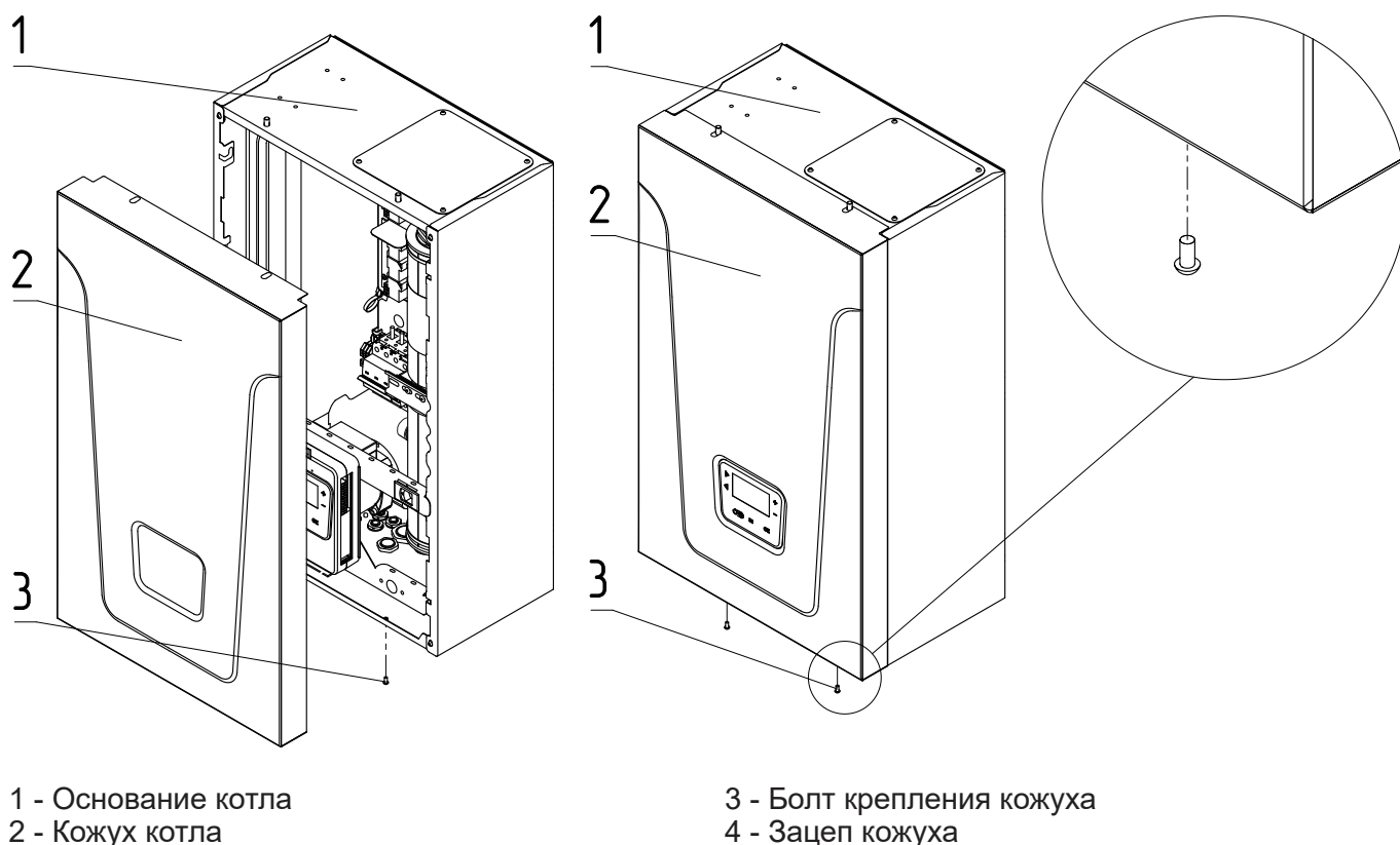
Рис.7 Снятие кожуха
