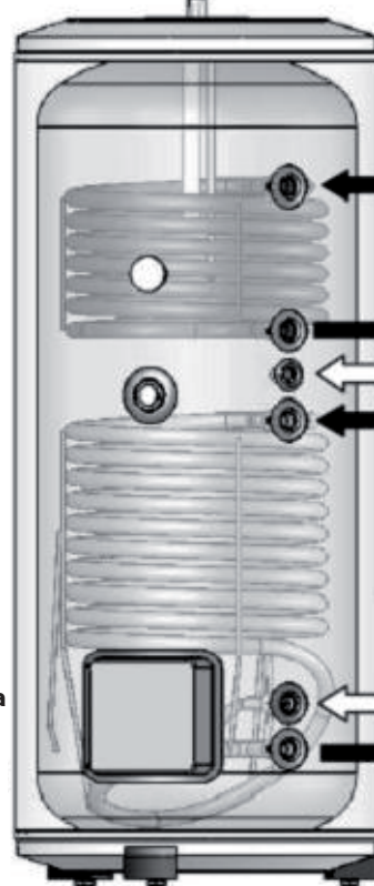
BOLLITORE 2S ↑ Uscita acqua calda
