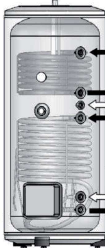
ACUMULADOR 2S Saída água quente
