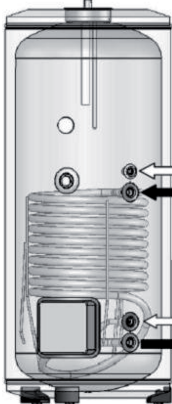
BOILER 1S ↑ Uitgang warm water
