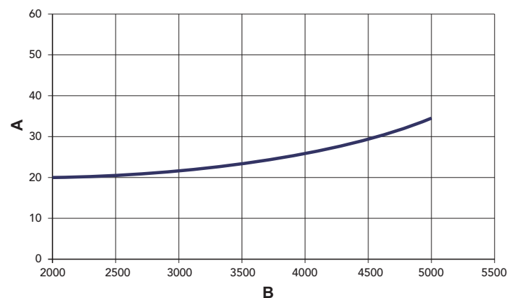
fig. 6 - Drukhoogteverlies
