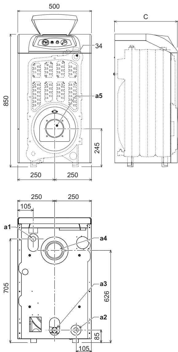
fig. 5 - Afmetingen, aansluitingen en hoofdcomponenten
