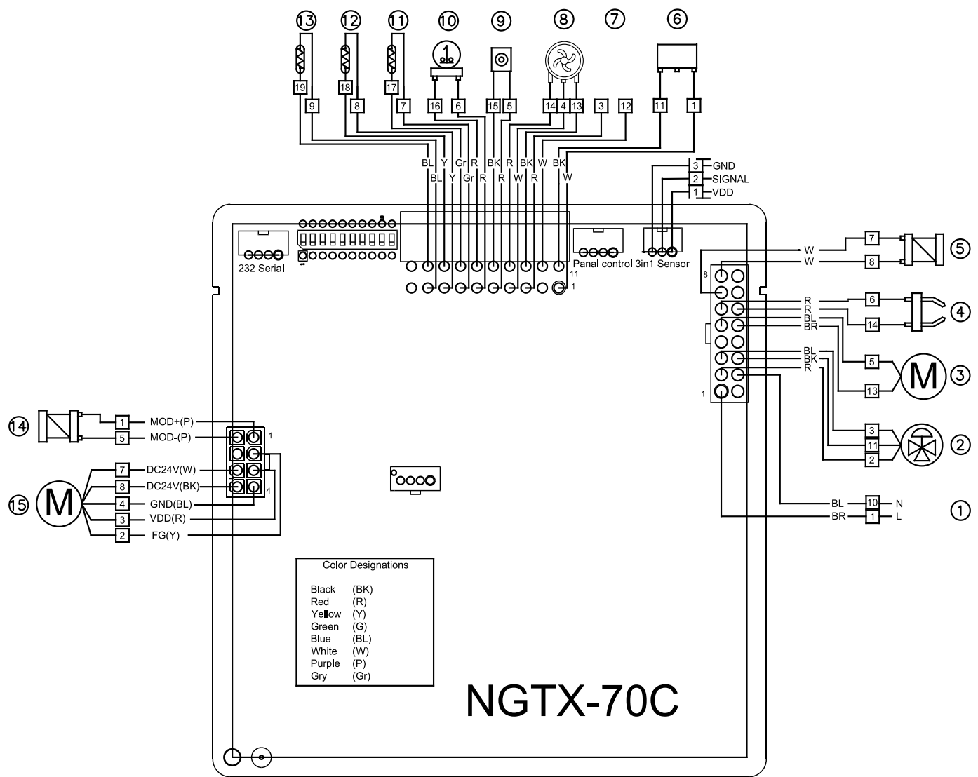
Рисунок 16. Схема электрическая.
