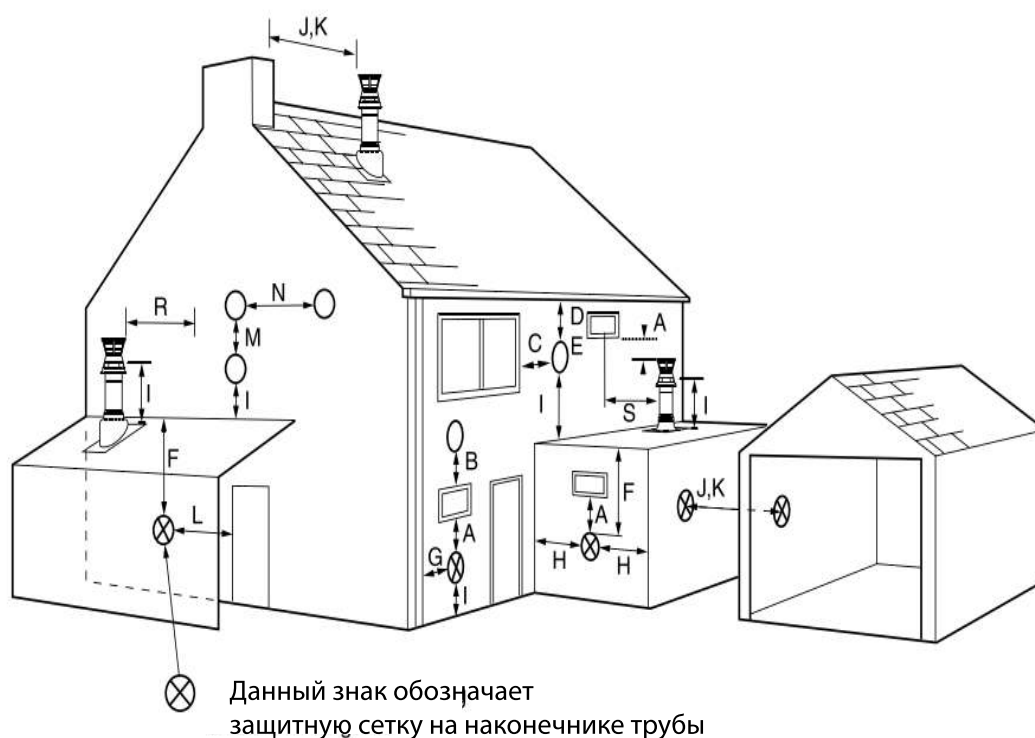
Рисунок 12. Рекомендуемые отступы дымохода.
