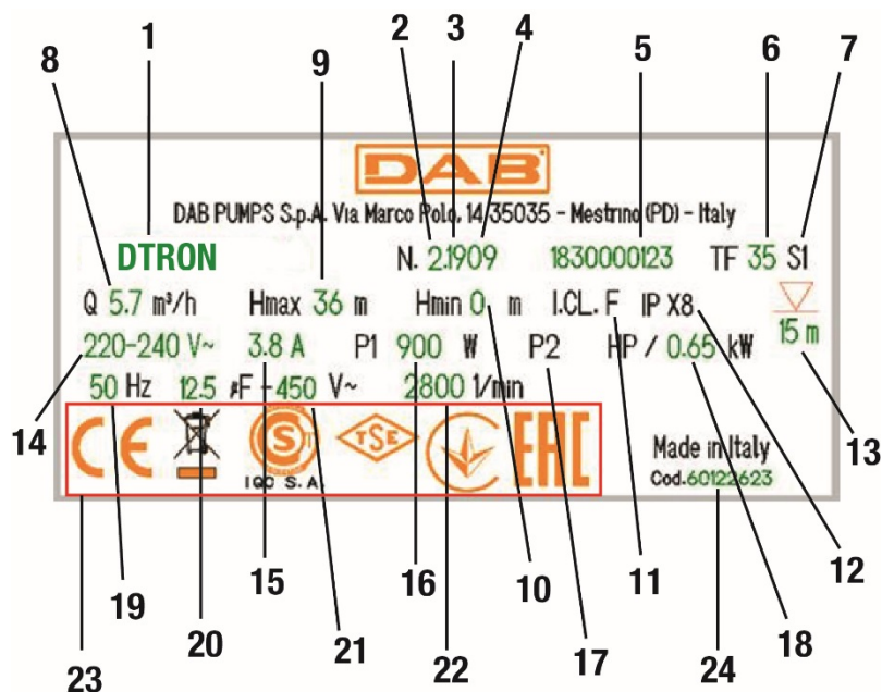
Obr.4 Štítek
