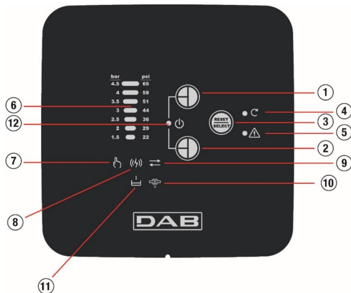
Figura 12: o painel do dispositivo COM BOX
