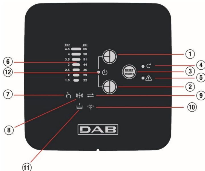
Рисунок 12: панель устройства COM BOX
