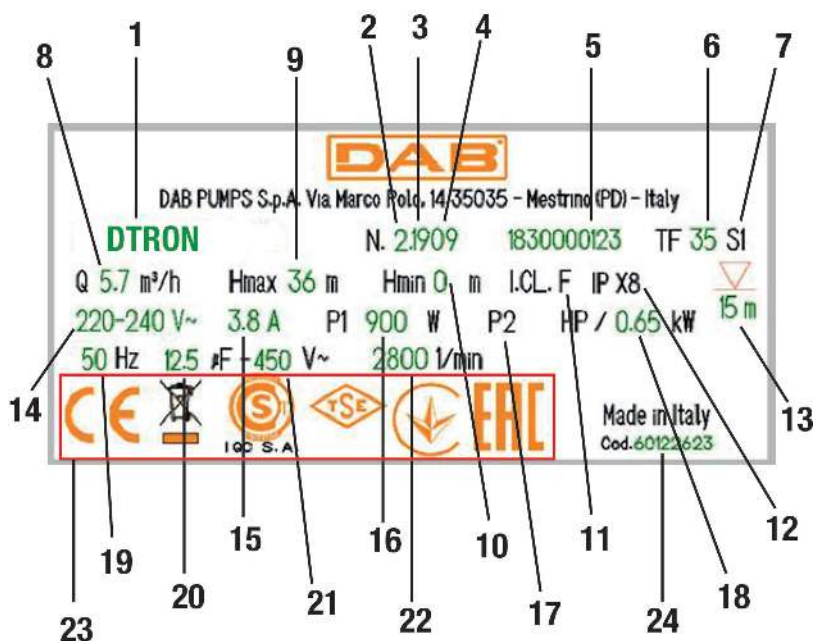
Fig.4 Eticheta tehnică
