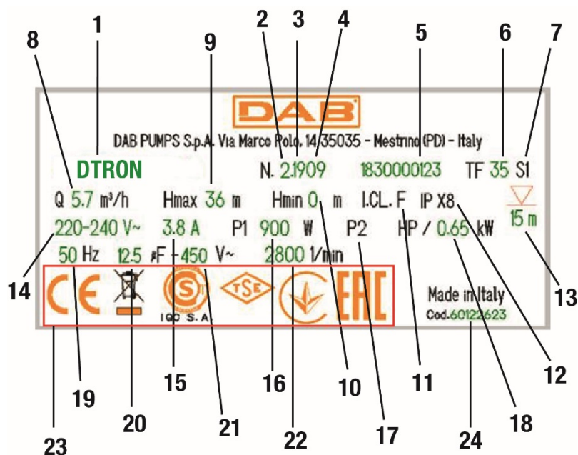
Фиг. 4 Табела
