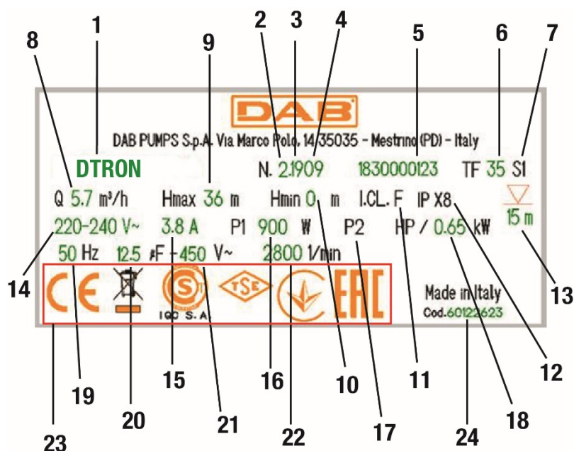
Εικ.4 Πινακίδα
