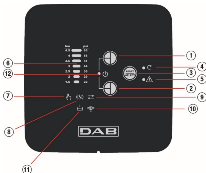
Фигура 12: Панелът на устройството COM BOX
