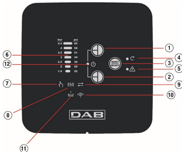
Rysunek 12: panel urządzenia COM BOX
