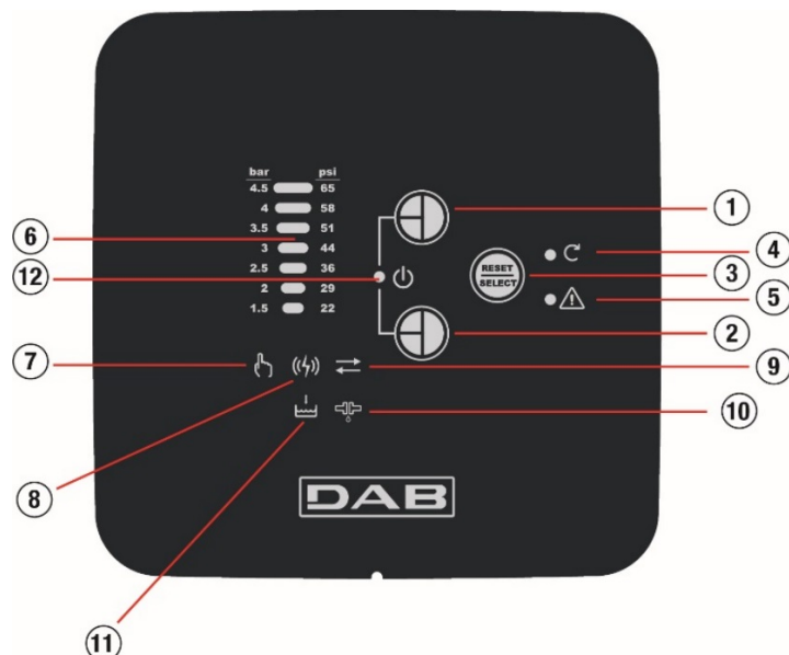
12. kép: COM BOX szerkezeti egység panelje
