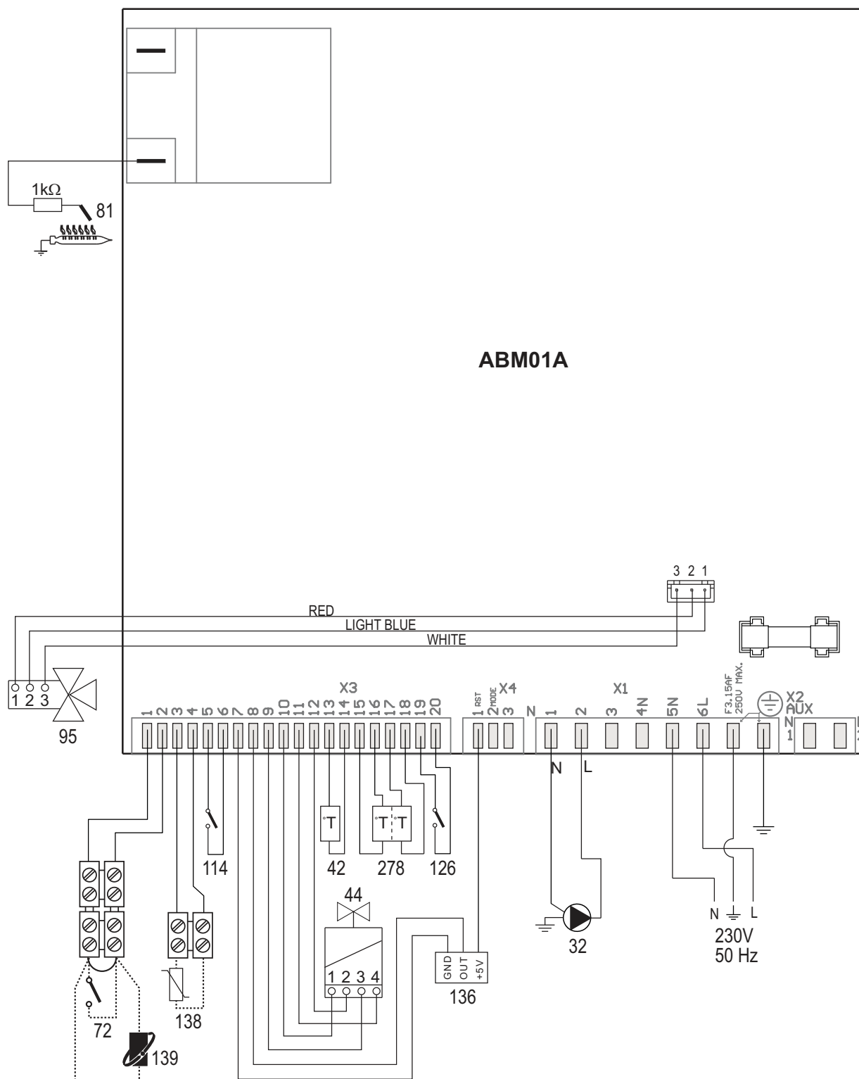
рис. 23- Электрическая схема
