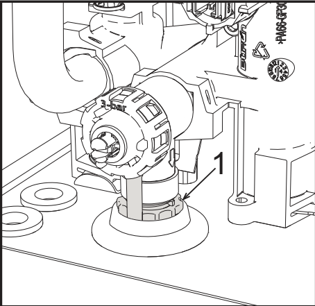
рис. 9- Предохранительный клапан со сливным краном
