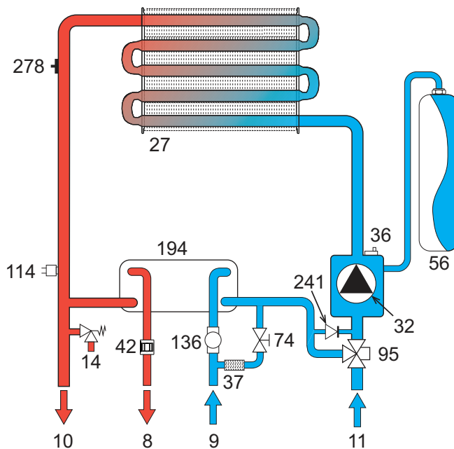
fig. 22- Circuit chauffage
