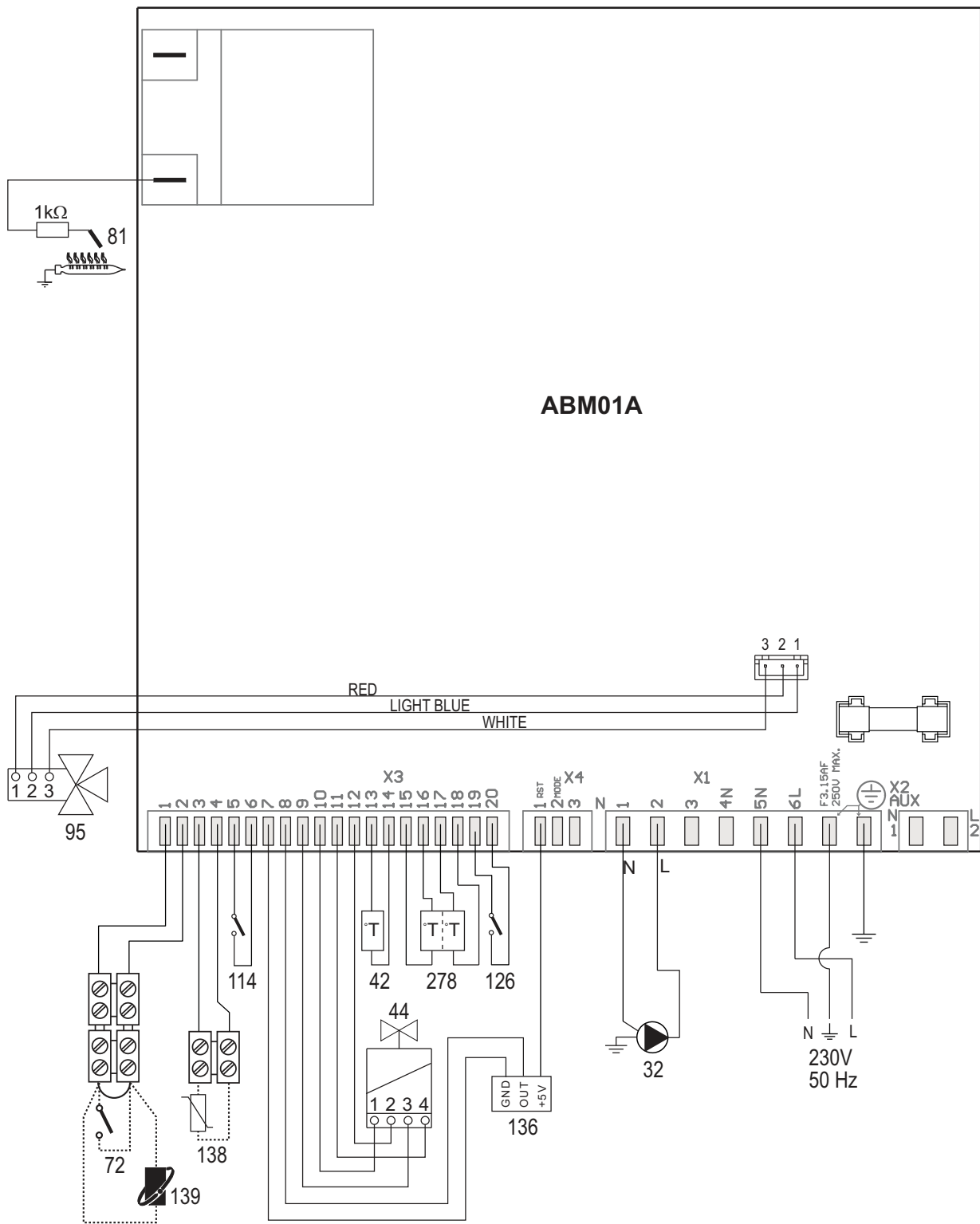
рис. 23- Электрическая схема
