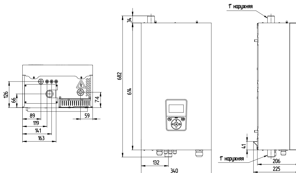
Рис.12 Габаритные размеры ZOTA SOLID-X 6-9 кВт
