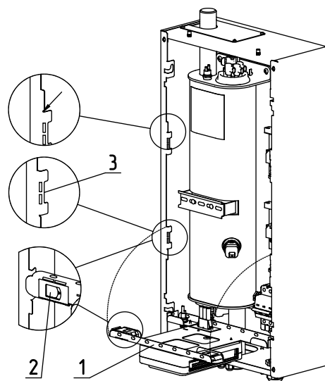
Рис.19 Откидывание кронштейна
