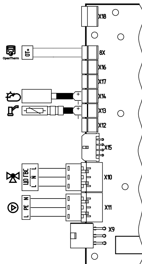
Рис.11 Подключение клапана приоритета бойлера ГВС, датчиков ГВС и улицы, и устройства OpenTherm к контроллеру «ZOTA X-Line 100E»
