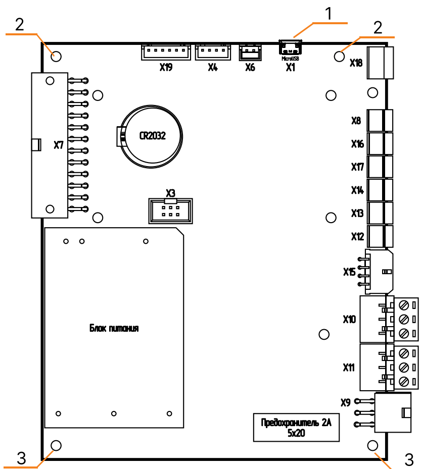
Рис.13 Плата контроллера
