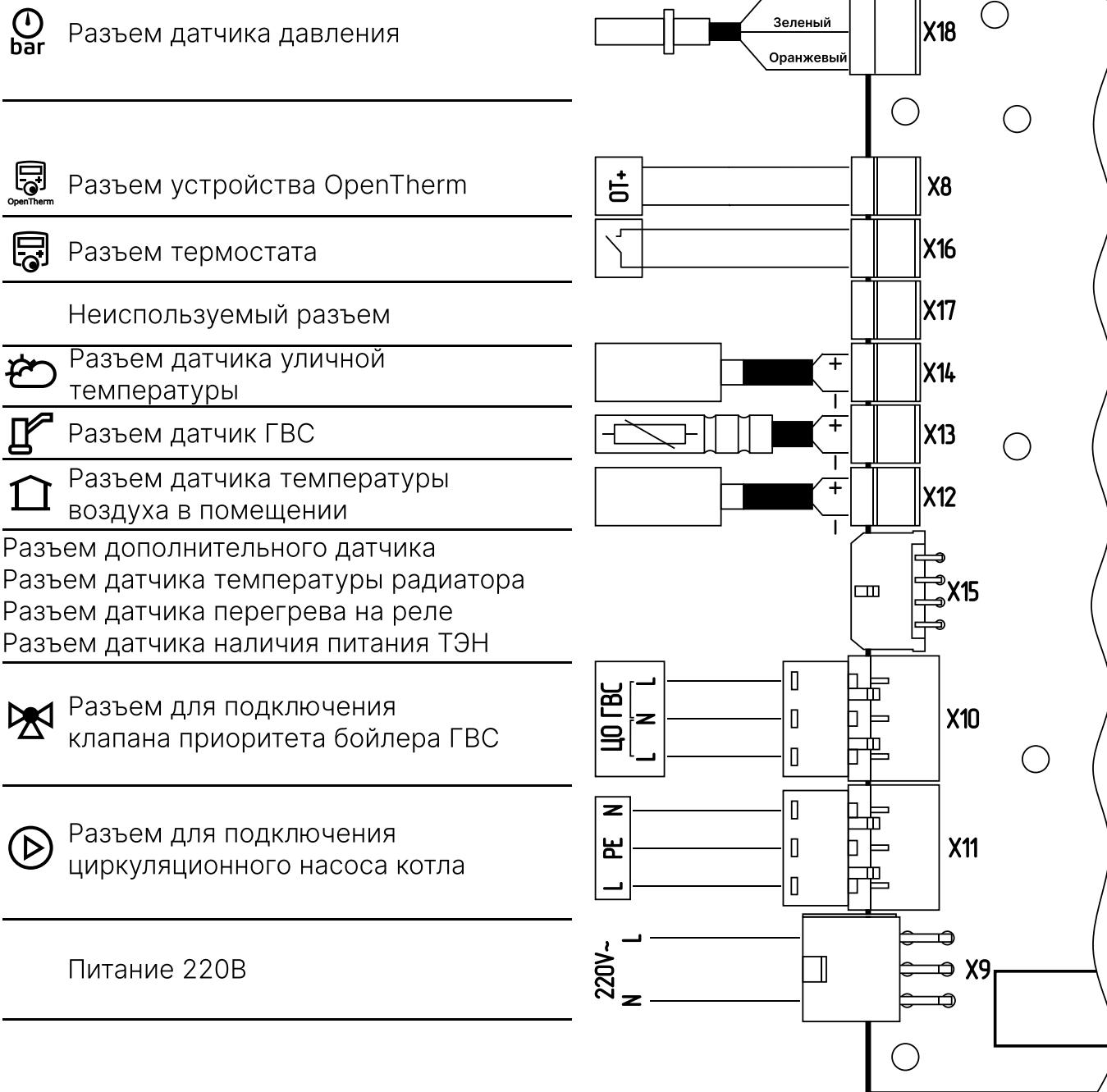
Рис.4 Схема подключения датчиков «ZOTA X-Line100E».
