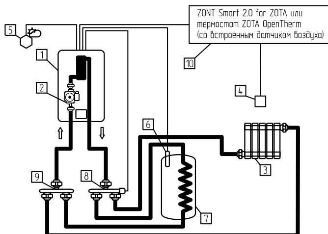
Термостат проводной ZOTA ZT-20H OT+
