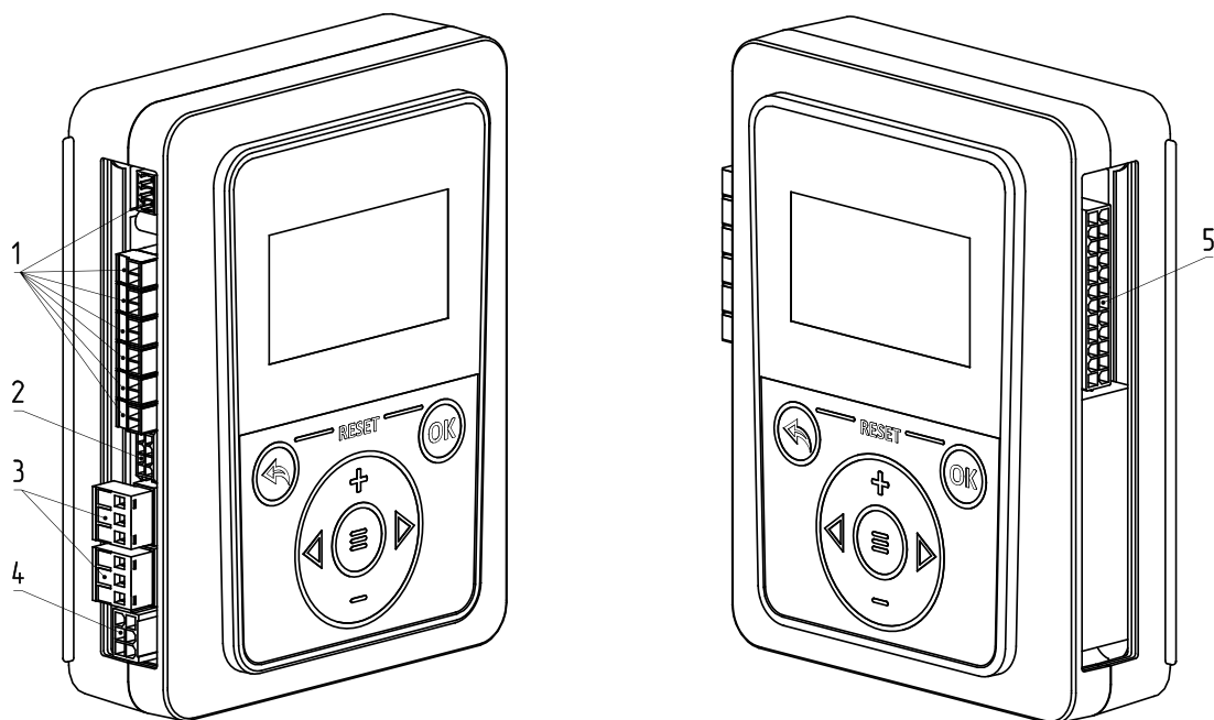
Рис.1 Корпус контроллера «ZOTA X-Line 100E»
