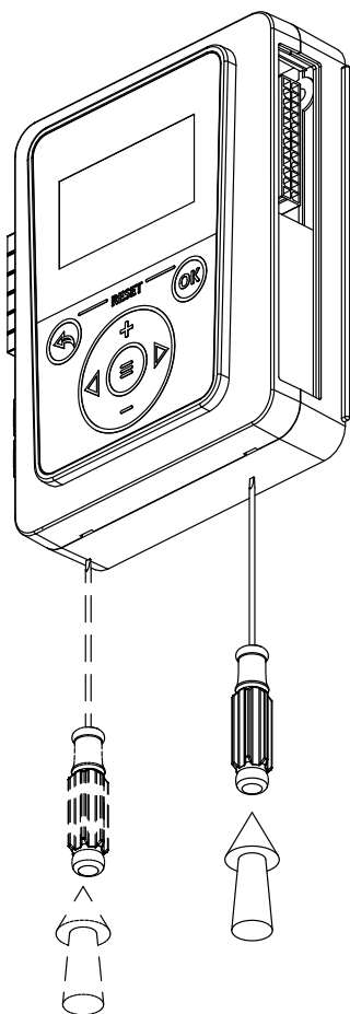
Рис.12 Демонтаж лицевой панели
