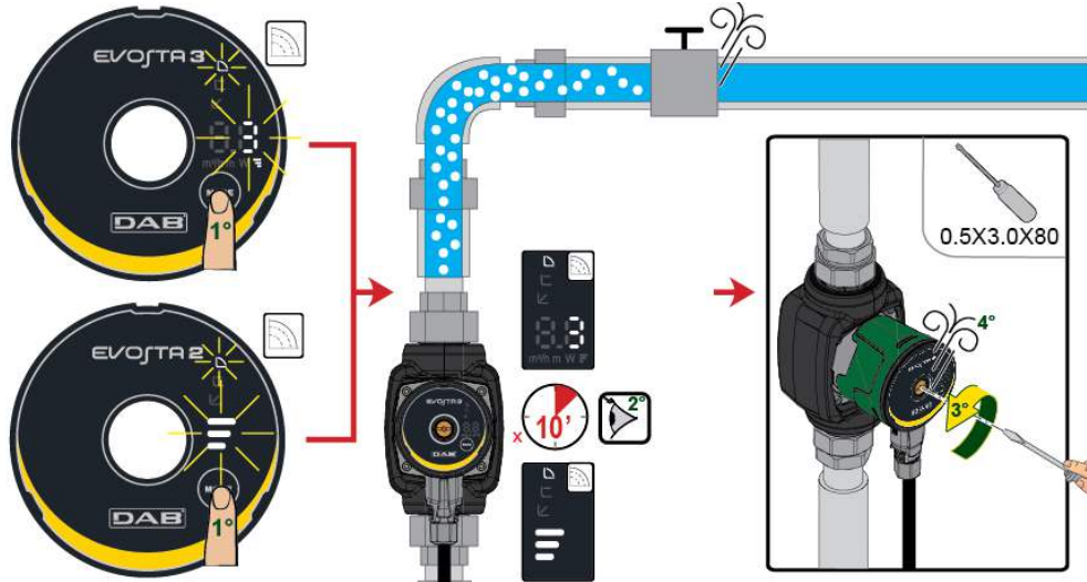
8 pav.: Oro išleidimas iš siurblio
