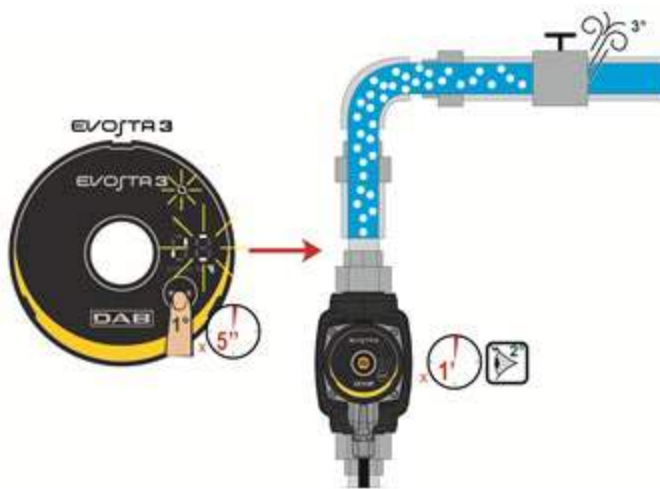
Малюнок 9: Автоматичний випуск газів з насоса
