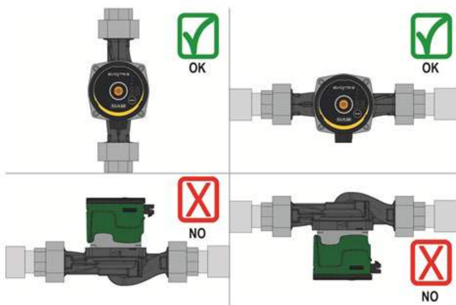
Abb. 3: Montageposition
