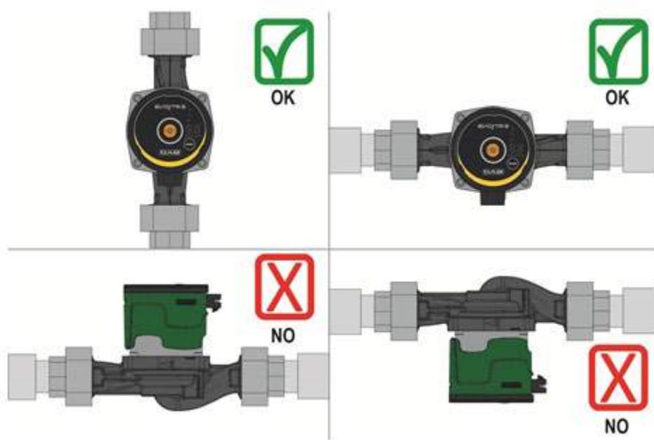
Εικόνα 3: Θέση συναρμολόγησης
