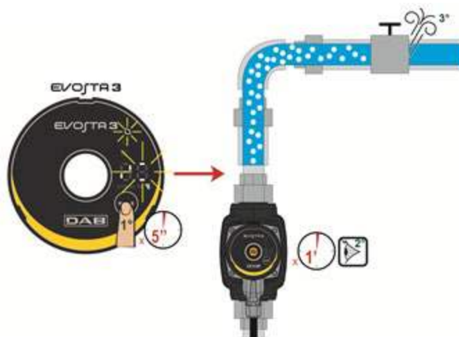
Abb. 9: Automatische Pumpenentlüftung
