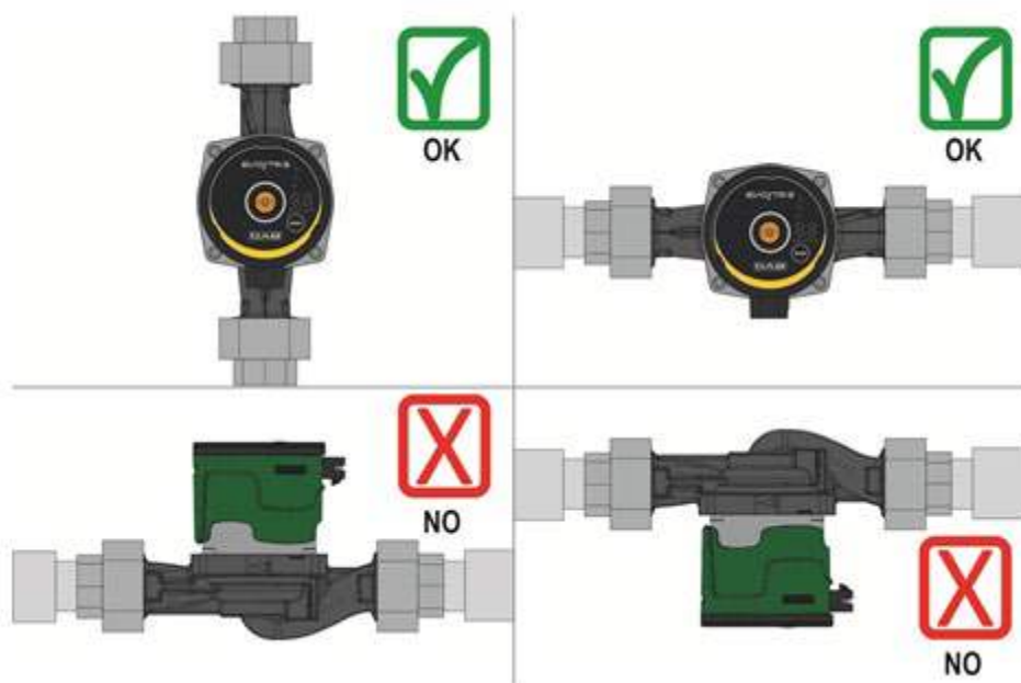
Afbeelding 3: montagepositie
