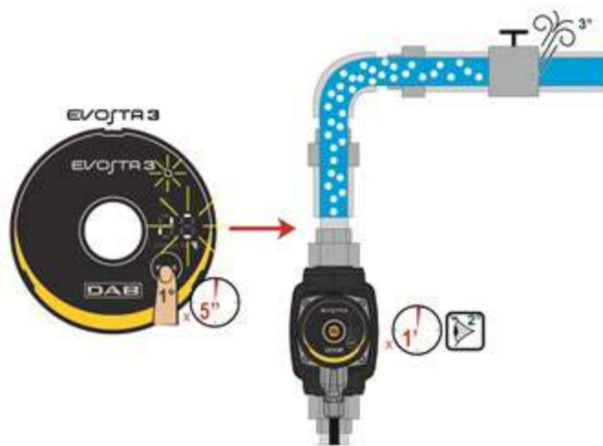
Figura 9: Aerisirea automată a pompei
