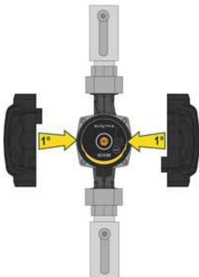
Рисунок 7: Изоляция корпуса насоса
