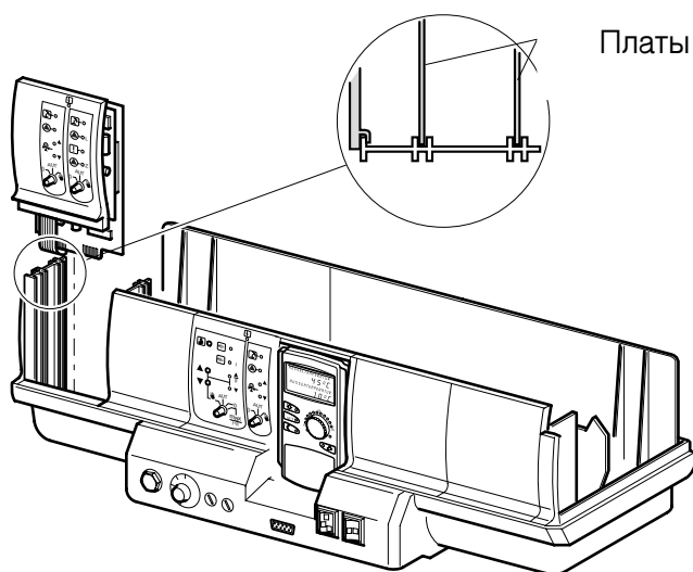
Рис. 4 Установка модуля
