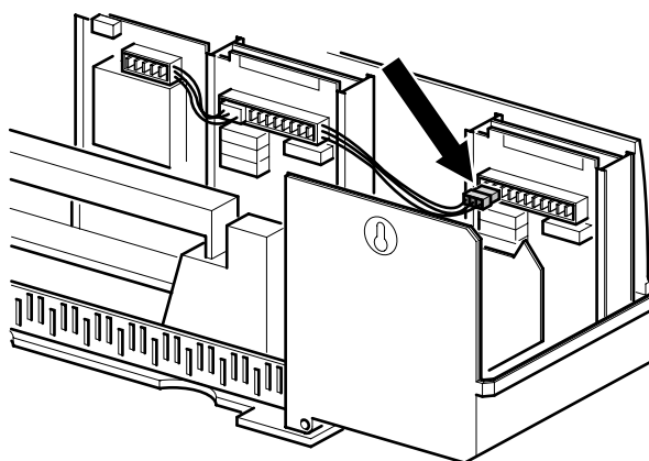
Рис. 5 Подключите напряжение
