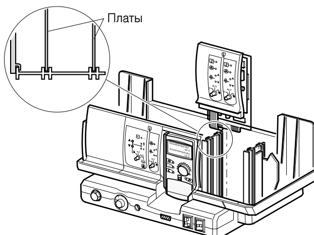
Рис. 4 Установка модуля
