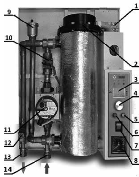
Рис.1 Устройство котла
