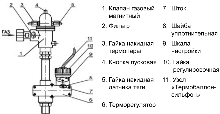
Рисунок 2. Блок автоматики
