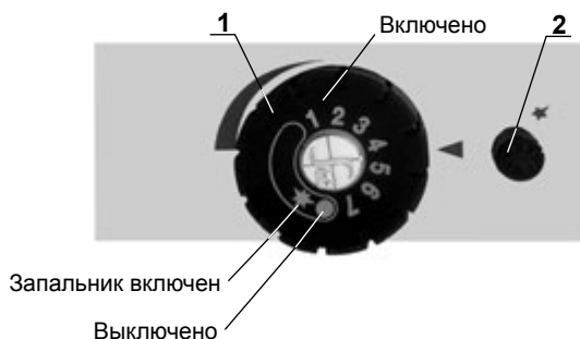
1. Ручка управления 2. Кнопка пьезорозжига
