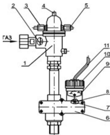
Рисунок 2. Блок автоматики
