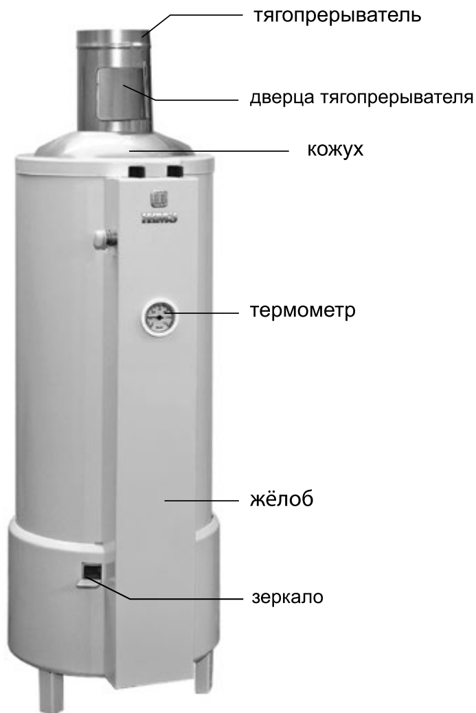
Рисунок 8. Аппарат Комфорт
