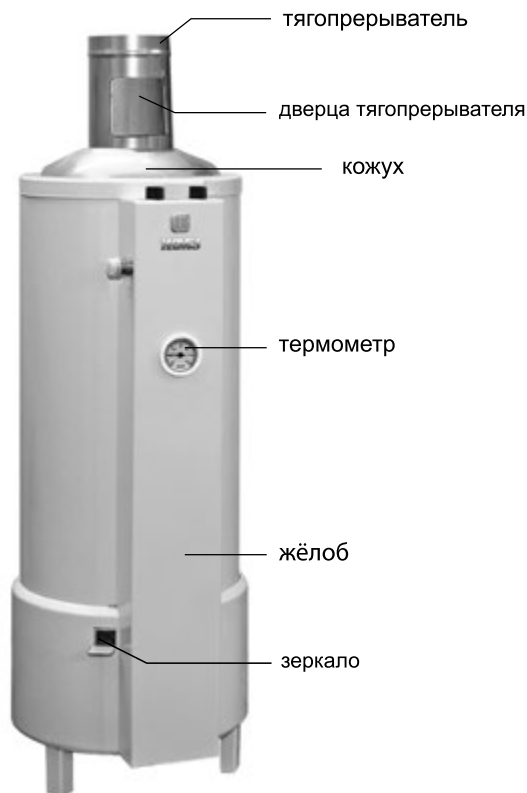
Рисунок 10. Аппарат Универсал
