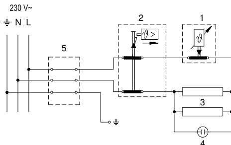
Instalația electrică
