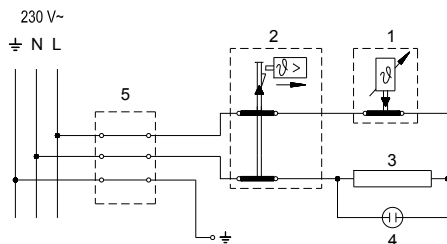
Электросхема
