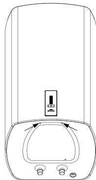
Fig. 4: Înlăturarea capacului protector
