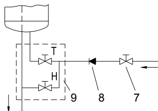
3 Сурет: Қысымсыз (ашық) жүйе
