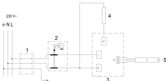
Рисунок 5: Электросхема
