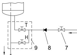
Рисунок 3: Безнапорная (открытая) система
