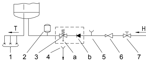
Рисунок 2: Напорная (закрытая) система
