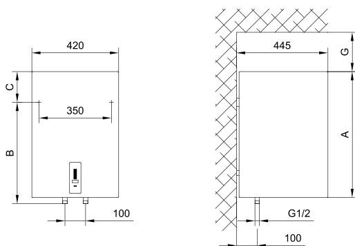
Рис. 1: Вертикальная установка на стену
