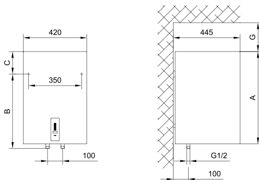
Fig. 1: Montarea verticală pe perete
