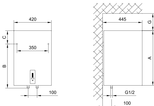
Мал. 1: Вертикальний монтаж на стіну
