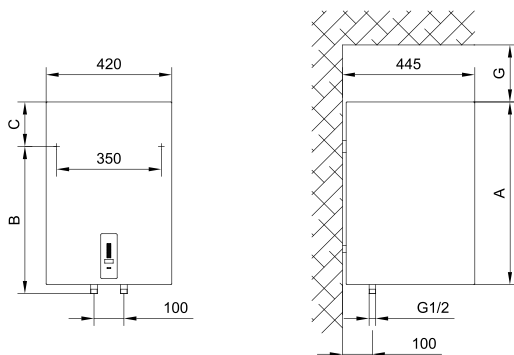
1 Сурет: Қабырғаға тігінен орнату
