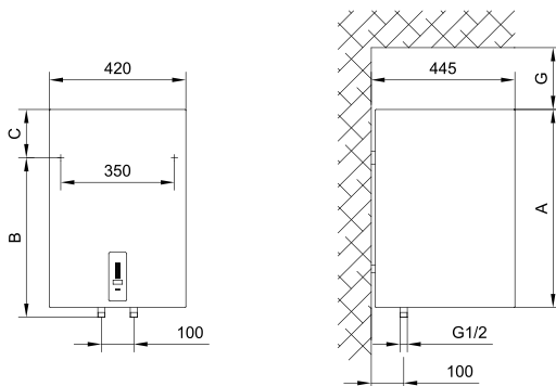
Sl. 1: Vertikalno montiranje na zid
