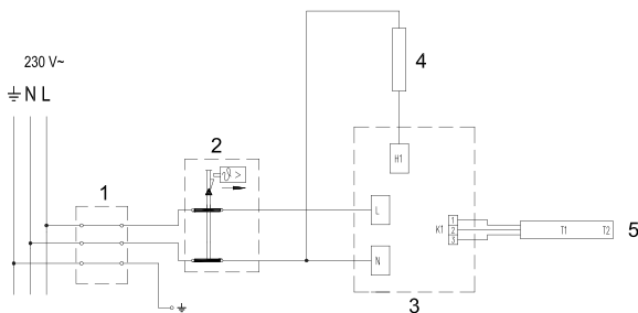
Fig. 5: Instalația electrică
