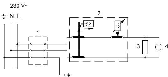
Электросхема
