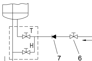
Открытая (проточная) система
