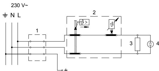
Электросхема
