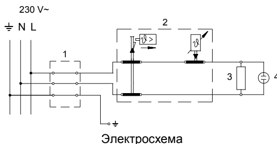
Электросхема
