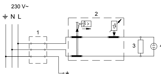
Электрсхемасы
