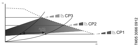
Рис. 21 Три кривые/настройки регулирования с постоянным давлением
