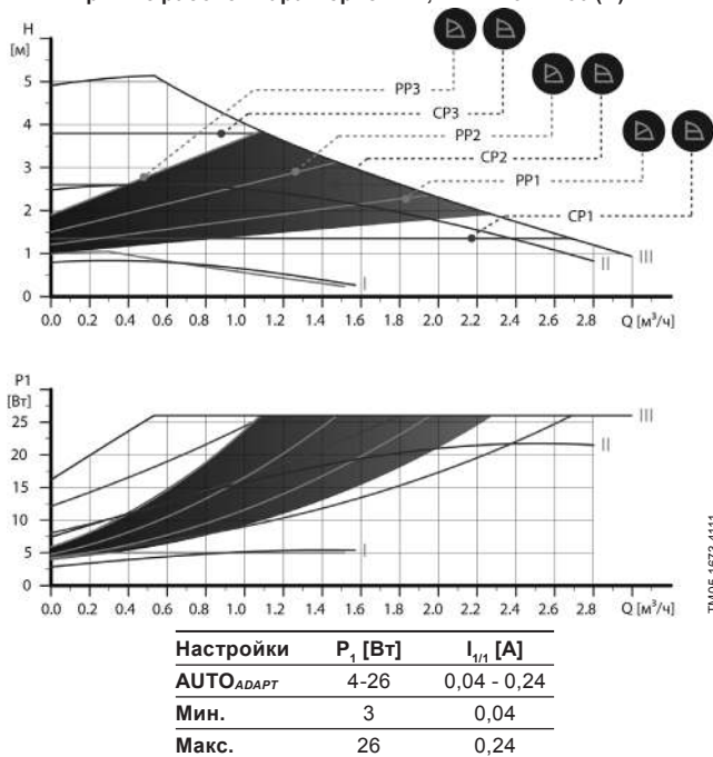
Рис. 33 ALPHA3 XX-50 (N)
