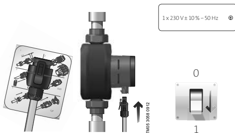
Рис. 10 Подключение к электросети
