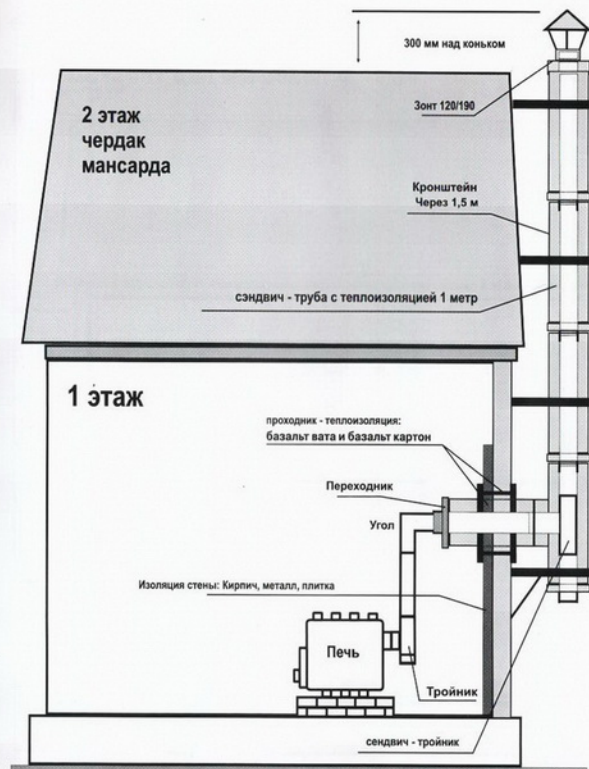
Рис. 3. УСТАНОВКА ПЕЧИ С НАРУЖНЕЙ СХЕМОЙ ДЫМОХОДА (СЭНДВИЧ)
