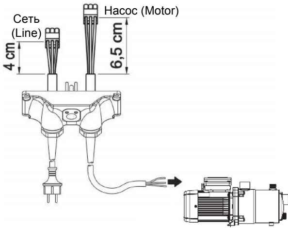
Рис. 2 Проводное подключение
