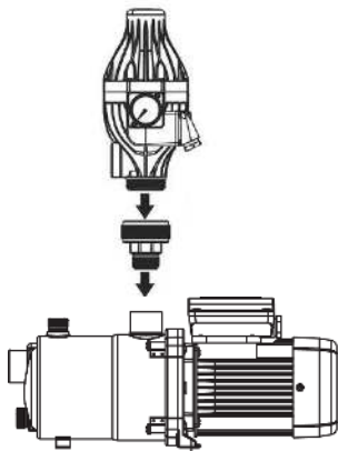
Рис. 1 Механическое подключение
